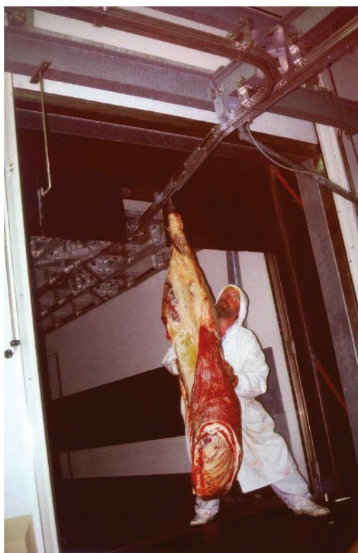
Photo 8.2. Exemple de dispositif de manutention (rail suspendu continu) intégré dans la conception des locaux et adapté au type de camion amené à accoster au quai pour assurer la continuité des manutentions à l'interface de transbordement.
