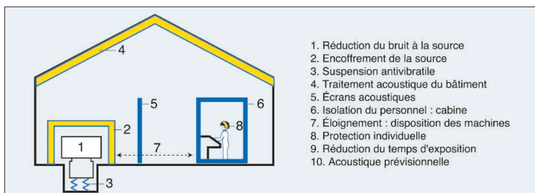
Figure 5.2. Différentes solutions d'insonorisation.
